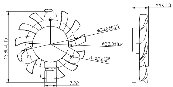
尺寸图 DIMENSIONS DRAWING
