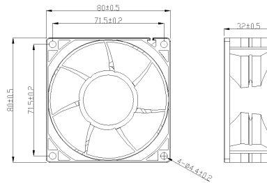
尺寸图 DIMENSIONS DRAWING
