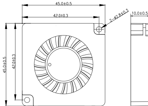
尺寸图 DIMENSIONS DRAWING
